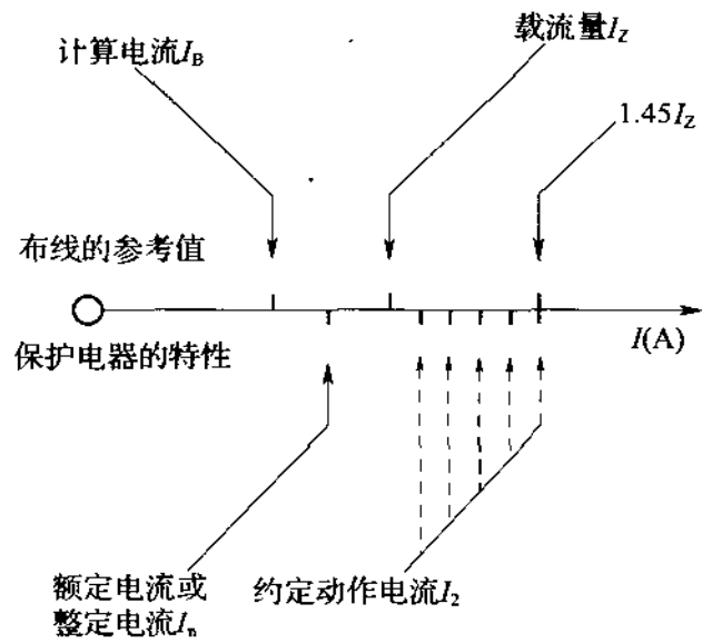
图 7 过电荷保护电器的动力特性关系图
